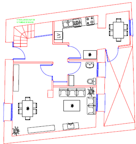
PLANTA BAJA
